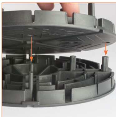
Les plots Multi et Multi+PLUS s'em-pilent les uns sur les autres, avec une rotation de 45° entre deux niveaux.
