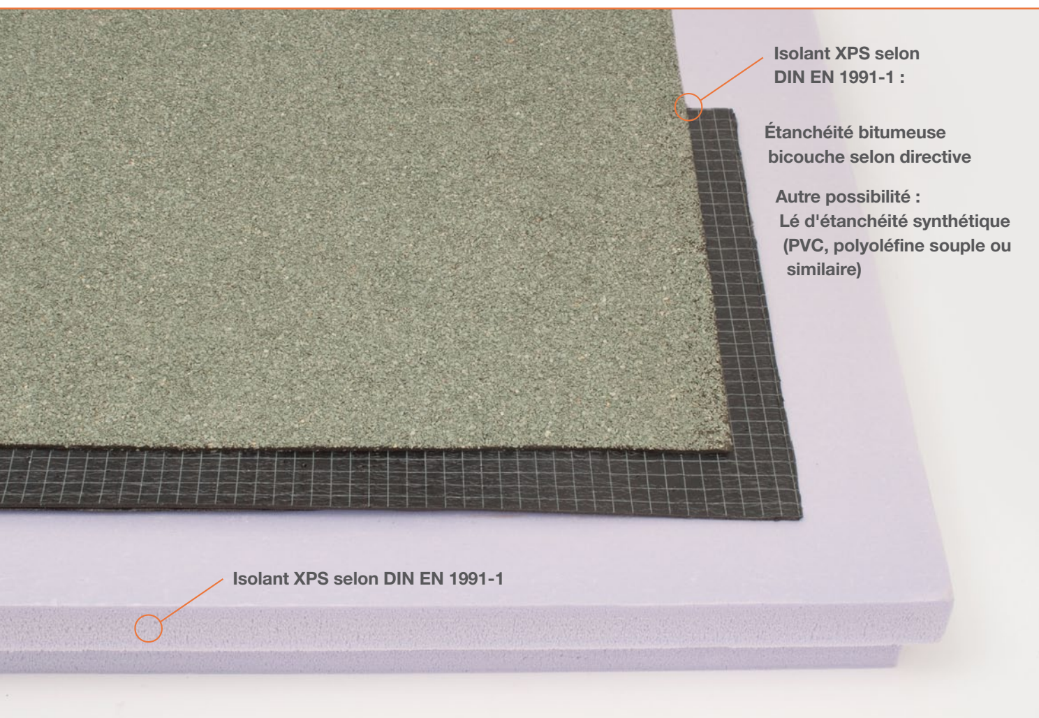
Isolation thermique XPS avec exemple d'étanchéité bitumeuse
